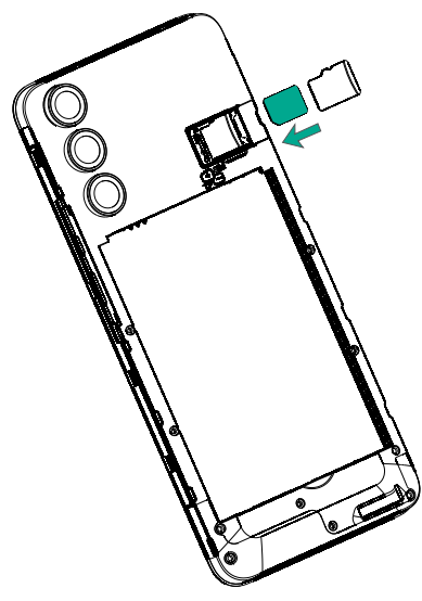
EN Insert SIM card(s)
